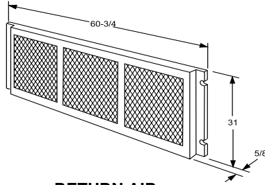
RETURN AIR GRILLE
